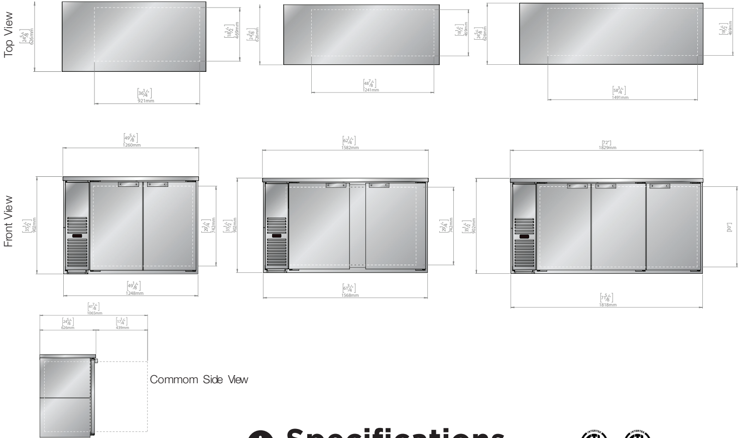
EBB-24-48G-B
